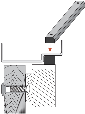
CX-DE1214-38 Barres d'écartement 3/8"
